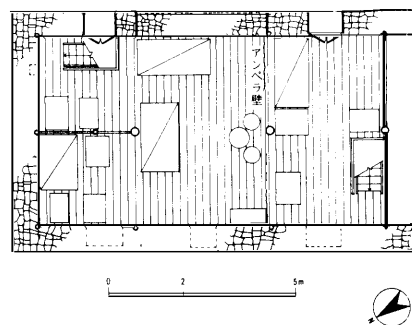
図19d No. 10主屋断面
