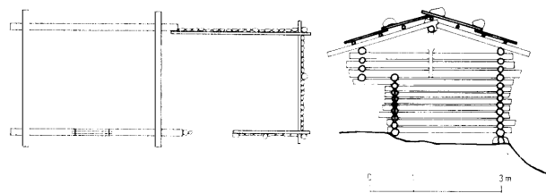
図9 当牛龍村・陶宅 (No. 4) 家畜小屋
