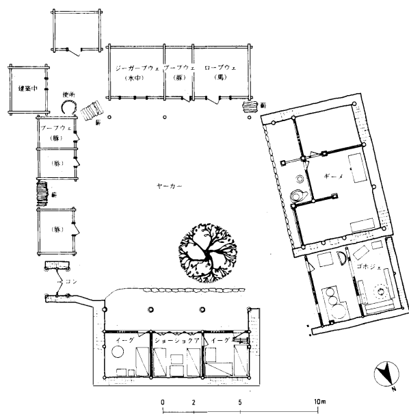
図13a 龍山郷四村・楊宅 (No. 6) 平面図
