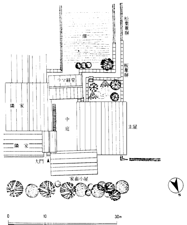
図18a 落水自然村クア家 (No. 9) 配置図
