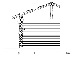
図4 b. 断面図
