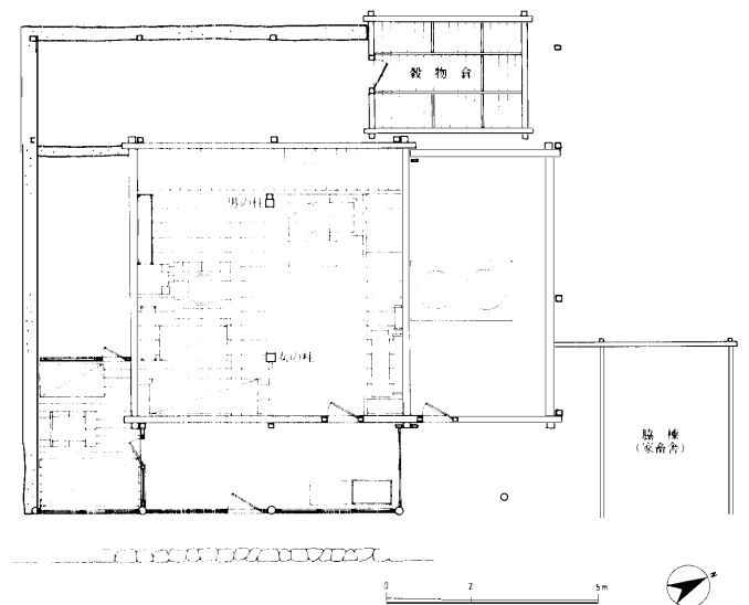
図18b 落水自然村クア家 (No. 9) 主屋平面図
