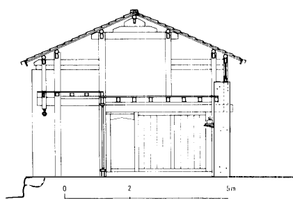
図8 c No. 4 南主屋断面図
