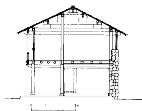
図11b No. 5 主屋断面図 (ターワークォ部分)
