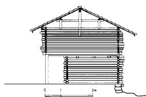
図13c No. 6 馬舎 (ローブウェ) 断面図
