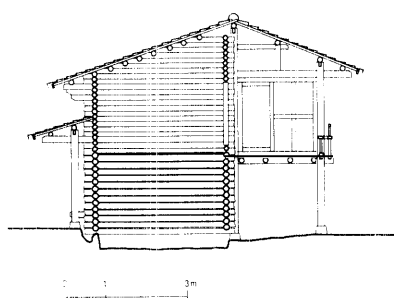
図16d No. 8 門屋断面図
