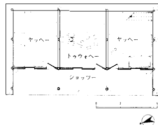
図6 a 大堂子村・紫有義氏宅 (No. 2) 1階平面
