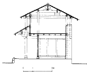
図13b No. 6 主屋断面図
