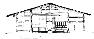
図16c No. 8 主屋断面図
