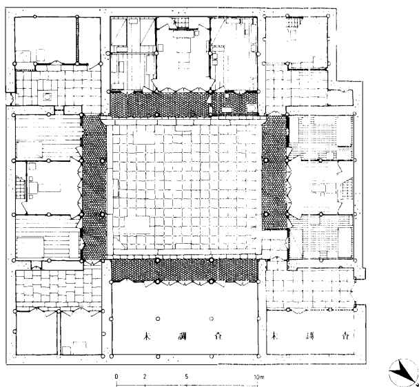
図20 喜洲鎮市戸街・張宅 (No. 11) 平面図
