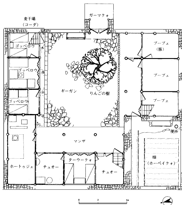
図11a 玉湖村李宅 (No. 5) 1階平面
