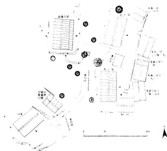
図8 a 龍山郷部当牛龍村・陶宅 (No. 4) 配置図
