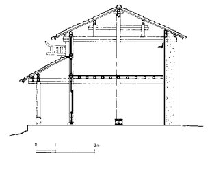
図6 b 断面図 (No. 2)
