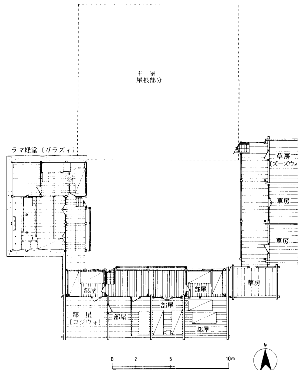
図16b No. 8 2階平面図
