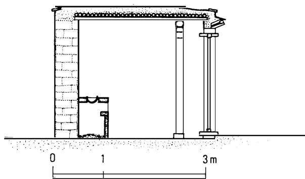
図21b No. 12 旧厨房部分断面図
