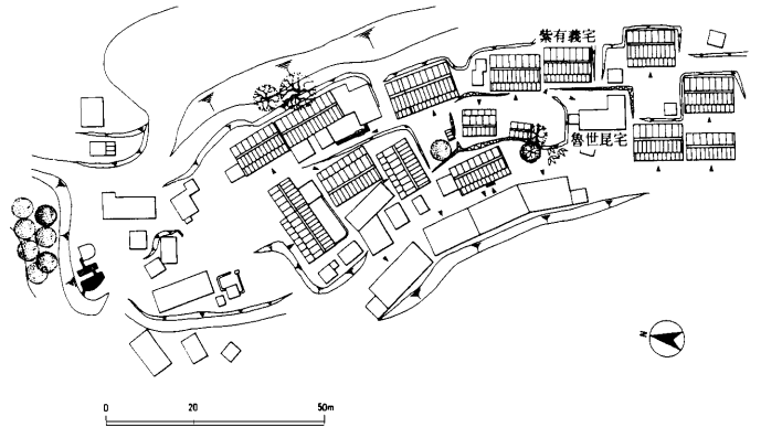
図5 南華県天申堂郷大堂子村・集落配置
