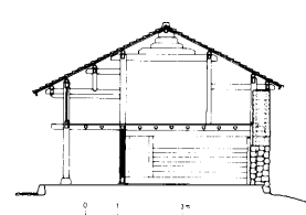
図11c No. 5 ブーブエ (家畜舎) 部分断面図
