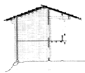
図18c No. 9 家畜舎断面図
