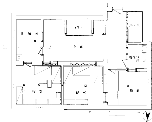
図21a ラサ市チョゴ村・シャマ宅 (No. 12) 平面図
