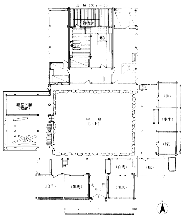
図16a 永寧ソナミ宅 (No. 8) 1階平面図
