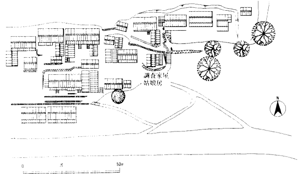
図3 南華県小岔河村・集落配置
